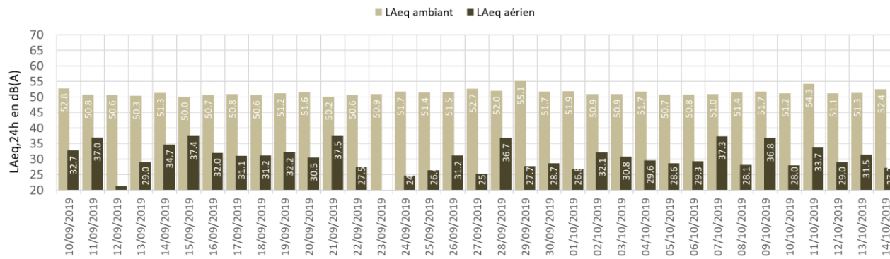
Évolution journalière du LAeq,24h - RUBELLES
