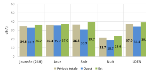
Rubelles - Indicateurs énergétiques moyens par périodes Dimanches
