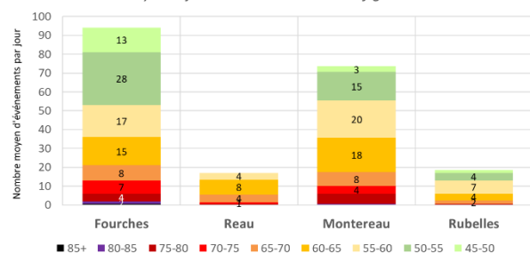
Distribution des L Max aéronefs sur la période de mesure Moyenne journalière - Samedis - Configuration EST
