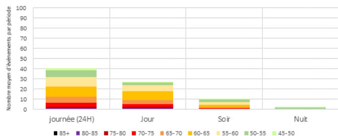
Distribution des LAmx - par périodes réglementaires - FOURCHES Tous jours confondus - Configuration Est
