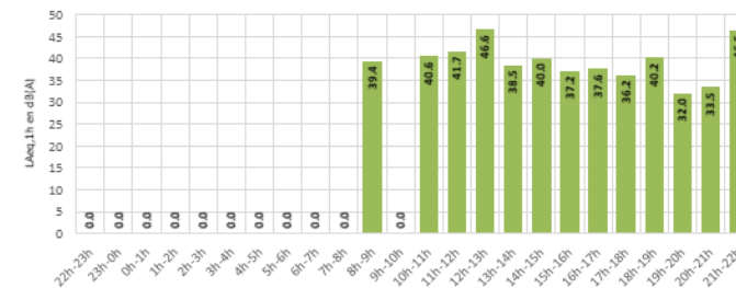
Distribution des LAMax - par périodes réglementaires - REAU Dimanches - Configuration Est
