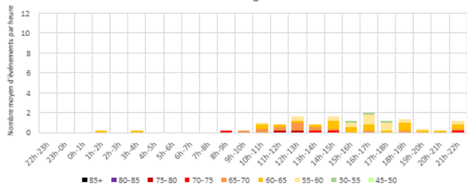
Distribution moyenne horaire des LAMax - REAU Samedis - Configuration Ouest
