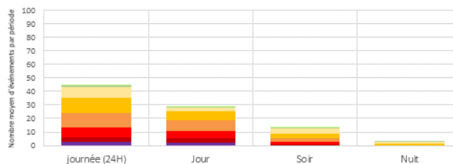
Distribution des SEL - par périodes réglementaires - FOURCHES Tous jours confondus - Toutes configurations
