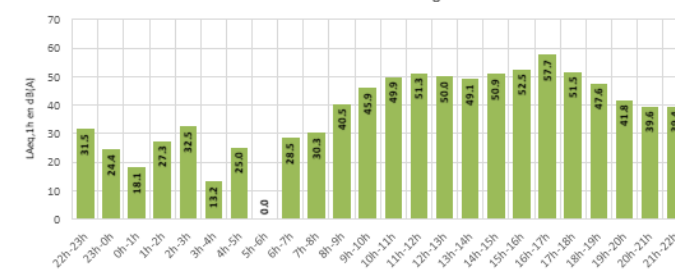
Distribution des LAmix - par périodes réglementaires - FOURCHES Jours ouvrables - Configuration Est
