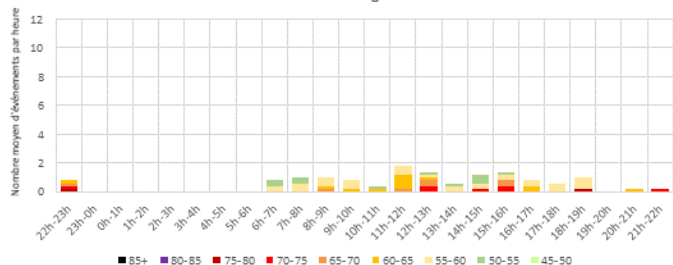
Distribution moyenne horaire des LAmx - REAU Dimanches - Configuration Ouest
