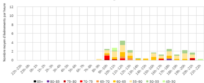
Distribution moyenne horaire des LAmx - MONTEREAU Dimanches - Configuration Est
