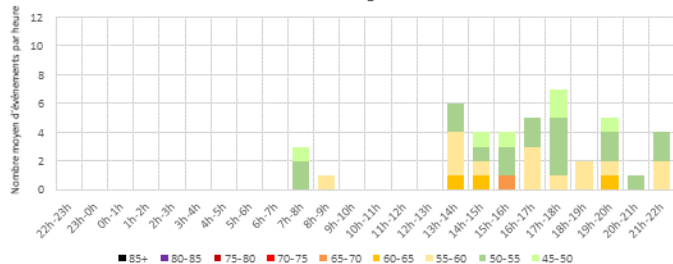
Distribution moyenne horaire des LAmx - MONTEREAU Dimanches - Configuration Est
