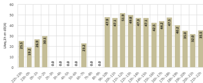
Niveau de bruit aérien - LAeq,1h - MONTEREAU Dimanches - Toutes configurations
