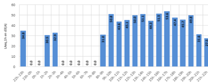
Distribution des LAMax - par périodes réglementaires - FOURCHES Dimanches - Configuration Ouest
