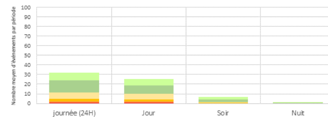
Distribution des émergences - par périodes réglementaires - MONTEREAU Tous jours confondus - Toutes configurations
