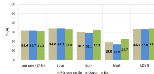
Rubelles - Indicateurs énergétiques moyens par périodes Samedis
