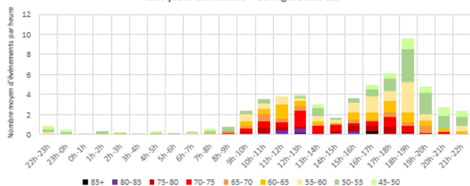
Distribution moyenne horaire des LAmax - FOURCHES Tous jours confondus - Configuration Est
