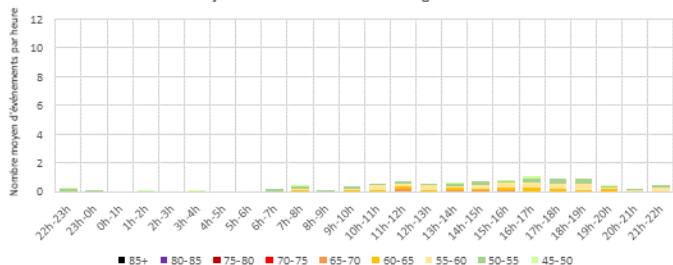
Distribution moyenne horaire des LAmax - RUBELLES Tous jours confondus - Configuration Ouest
