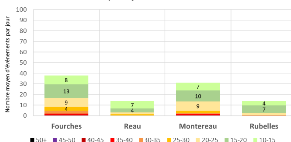
Distribution des émergences sur la période de mesure Moyenne journalière - Dimanches
