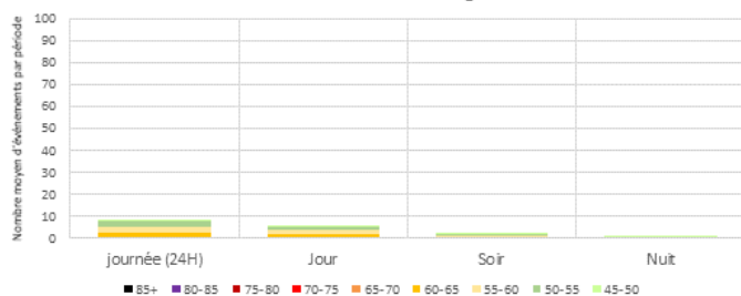
Distribution des LAmax - par périodes réglementaires - RUBELLES Jours ouvrables - Configuration Ouest
