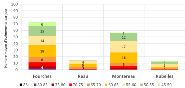
Distribution des L Max aéronefs sur la période de mesure Moyenne journalière - Samedis
