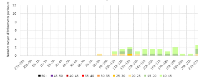
Distribution moyenne horaire des émergences - REAU Samedis - Configuration Est
