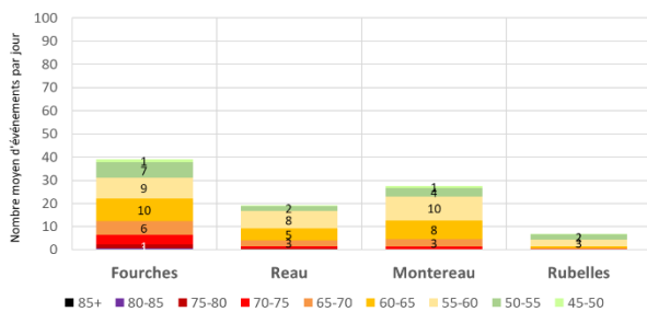
Distribution des L Max aéronefs sur la période de mesure Moyenne journalière - Jours ouvrables Configuration OUEST
