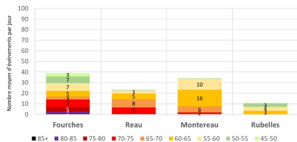
Distribution des L Max aéronefs sur la période de mesure Moyenne journalière - Jours ouvrables Configuration EST
