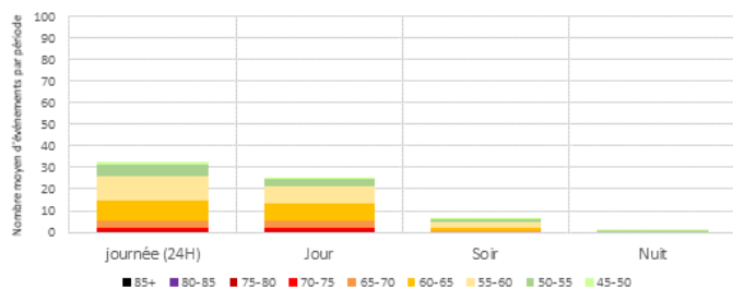
Distribution des LAmax - par périodes réglementaires - MONTEREAU Tous jours confondus - Configuration Ouest
