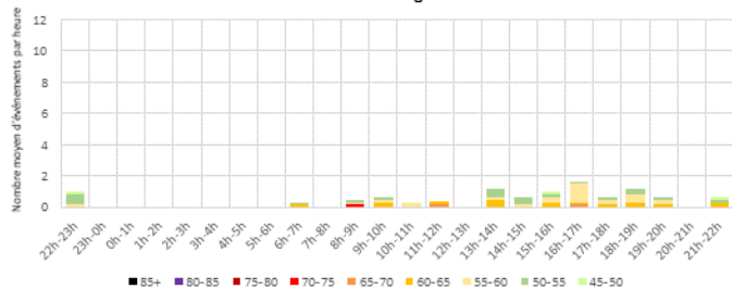
Distribution des LAmx - par périodes réglementaires - RUBELLES Jours ouvrables - Configuration Est
