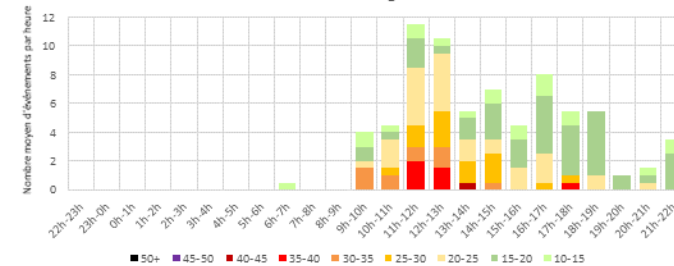
Distribution moyenne horaire des émergences - MONTEREAU Samedis - Configuration Est
