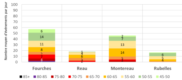
Distribution des L Max aéronefs sur la période de mesure Moyenne journalière - Tous types de jours confondus - Configuration EST
