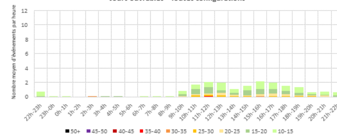
Distribution moyenne horaire des émergences - REAU Jours ouvrables - Configuration Ouest
