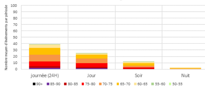
Distribution des SEL - par périodes réglementaires - FOURCHES Jours ouvrables - Configuration Est
