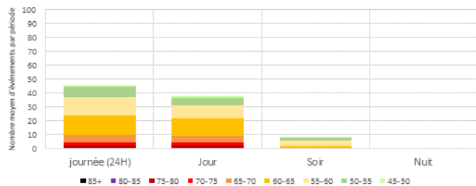
Distribution des LAmax - par périodes réglementaires - MONTEREAU Tous jours confondus - Configuration Est
