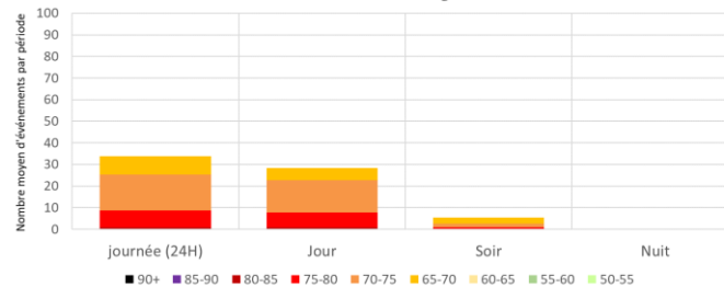
Distribution des SEL - par périodes réglementaires - MONTEREAU Jours ouvrables - Configuration Est
