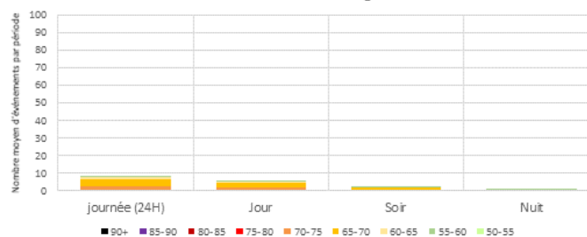
Distribution des SEL - par périodes réglementaires - RUBELLES Jours ouvrables - Configuration Ouest
