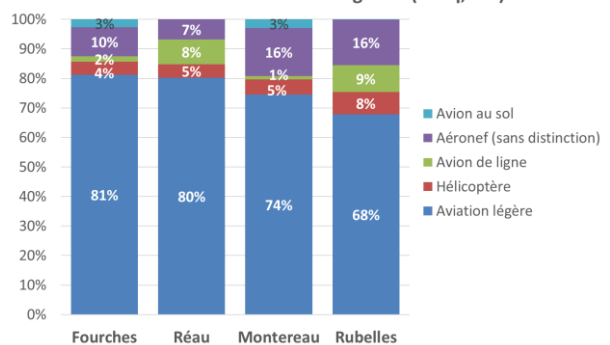
Contribution sonore énergétique de chaque type d'aéronef dans le bruit aérien global (LAeq,24h)
