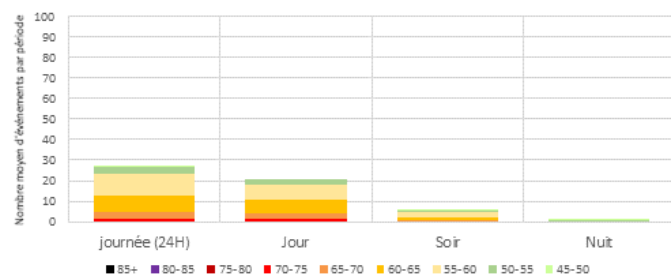
Distribution des LAmx - par périodes réglementaires - MONTEREAU Jours ouvrables - Configuration Est
