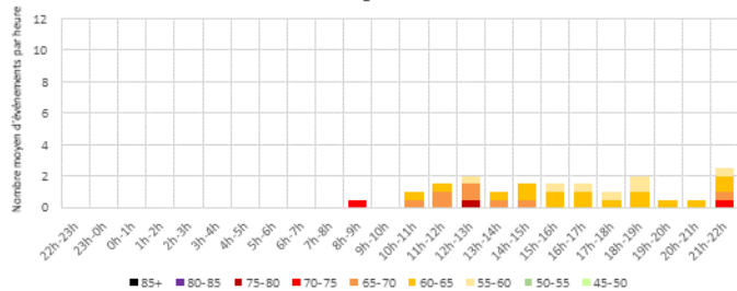
Distribution moyenne horaire des LAMax - REAU Samedis - Configuration Est
