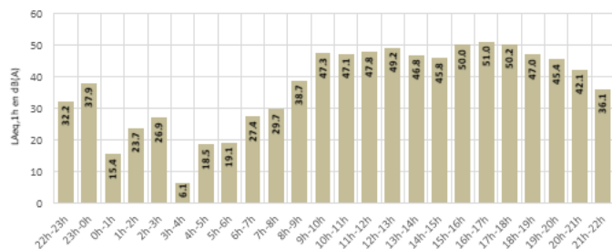
Niveau de bruit aérien - LAeq,1h - FOURCHES Tous jours confondus - Toutes configurations
