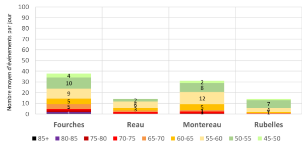
Distribution des L Max aéronefs sur la période de mesure Moyenne journalière - Dimanches
