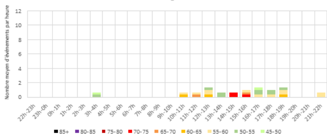
Distribution moyenne horaire des LAMax - RUBELLES Samedis - Configuration Est
