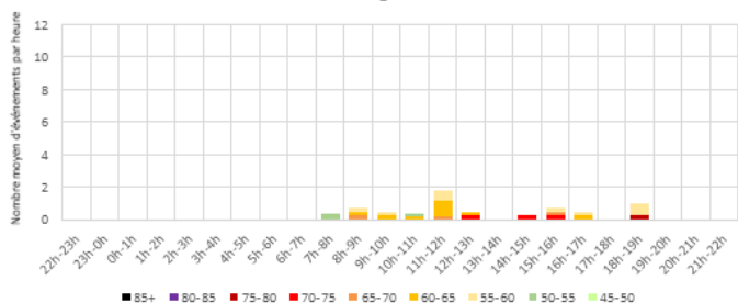
Distribution moyenne horaire des LAmx - REAU Dimanches - Configuration Est
