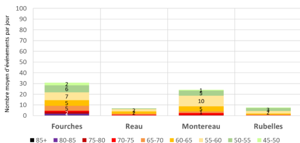
Distribution des L Max aéronefs sur la période de mesure Moyenne journalière - Dimanches - Configuration OUEST
