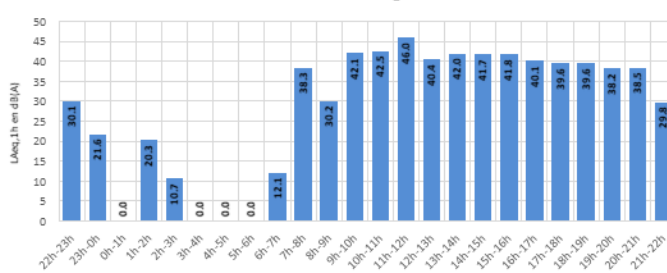
Niveau de bruit aérien - LAeq,1h - MONTEREAU Jours ouvrables - Configuration Ouest
