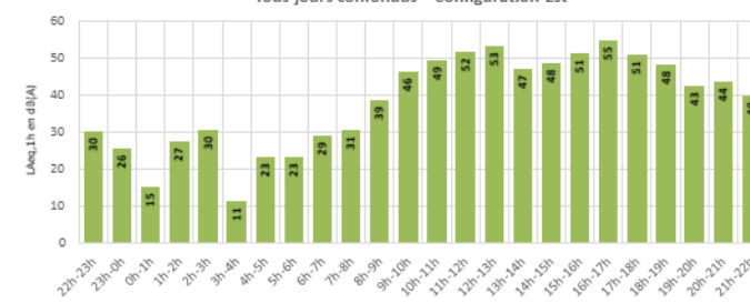
Niveau de bruit aérien - LAeq,1h - FOURCHES Tous jours confondus - Configuration Est
