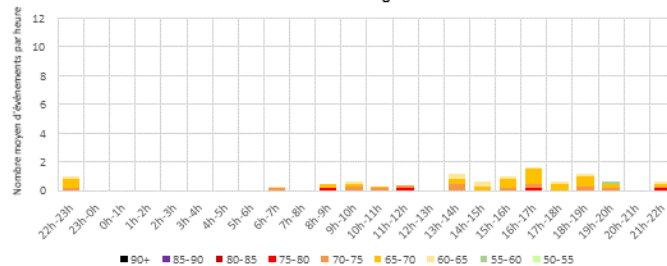
Distribution des SEL - par périodes réglementaires - RUBELLES Jours ouvrables - Configuration Est
