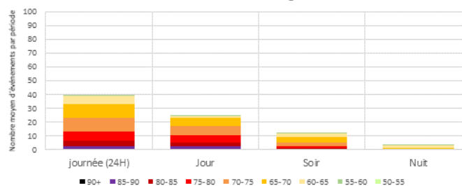
Distribution des SEL - par périodes réglementaires - FOURCHES Jours ouvrables - Configuration Ouest
