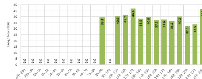
Distribution des LAMax - par périodes réglementaires - REAU Samedis - Configuration Est
