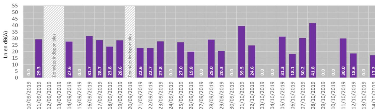
Évolution journalière du Ln aérien - FOURCHES
