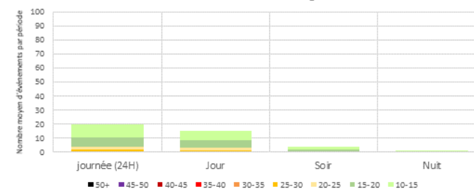
Distribution des émergences - par périodes réglementaires - REAU Jours ouvrables - Configuration Ouest
