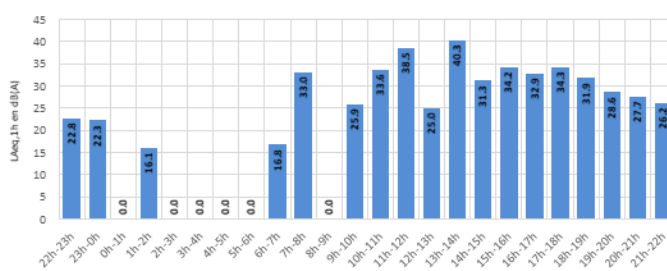
Niveau de bruit aérien - LAeq,1h - RUBELLES Jours ouvrables - Configuration Ouest
