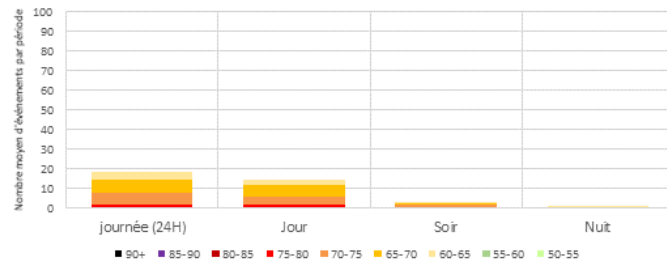
Distribution des SEL - par périodes réglementaires - RUBELLES Samedis - Configuration Est
