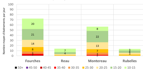
Distribution des émergences sur la période de mesure Moyenne journalière - Samedis
