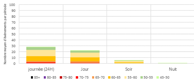
Distribution des LAmax - par périodes réglementaires - MONTEREAU Tous jours confondus - Configuration Est
