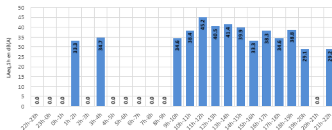
Distribution des LAMax - par périodes réglementaires - REAU Samedis - Configuration Ouest
