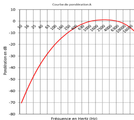
Filter de pondération A
