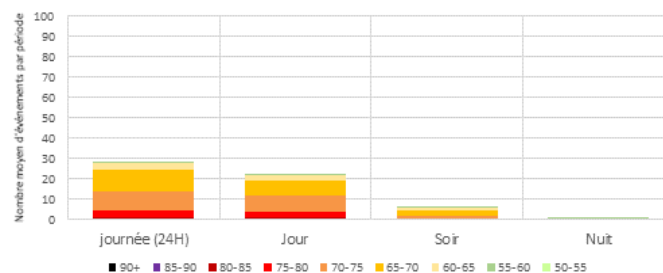
Distribution des SEL - par périodes réglementaires - MONTEREAU Tous jours confondus - Configuration Est
