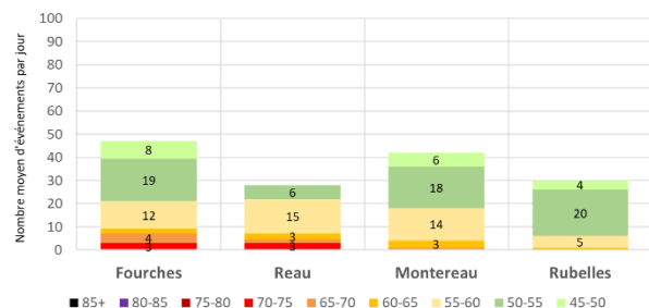
Distribution des L Max aéronefs sur la période de mesure Moyenne journalière - Dimanches - Configuration EST
