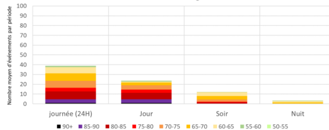
Distribution des SEL - par périodes réglementaires - FOURCHES Jours ouvrables - Configuration Est
