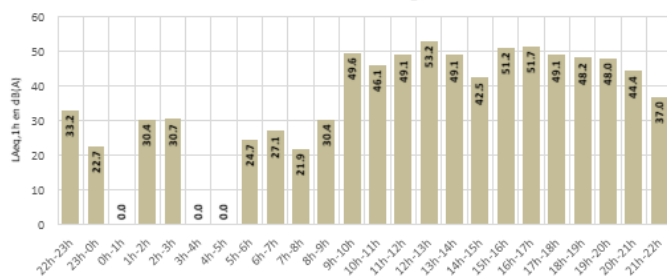
Niveau de bruit aérien - LAeq,1h - FOURCHES Samedis - Toutes configurations
