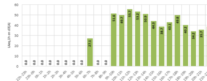
Distribution des LAMax - par périodes réglementaires - MONTEREAU Samedis - Configuration Est
