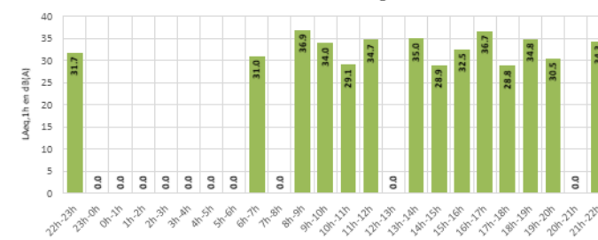
Distribution des LAMax - par périodes réglementaires - RUBELLES Jours ouvrables - Configuration Est
