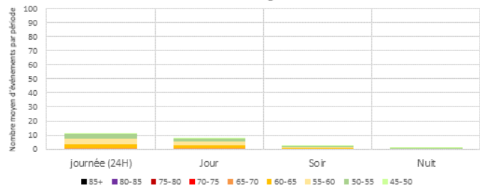
Distribution des LAmx - par périodes réglementaires - RUBELLES Samedis - Configuration Est
