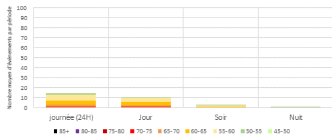
Distribution des LAmax - par périodes réglementaires - REAU Tous jours confondus - Configuration Est
