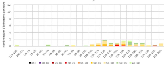
Distribution moyenne horaire des LAMax - RUBELLES Samedis - Configuration Ouest
