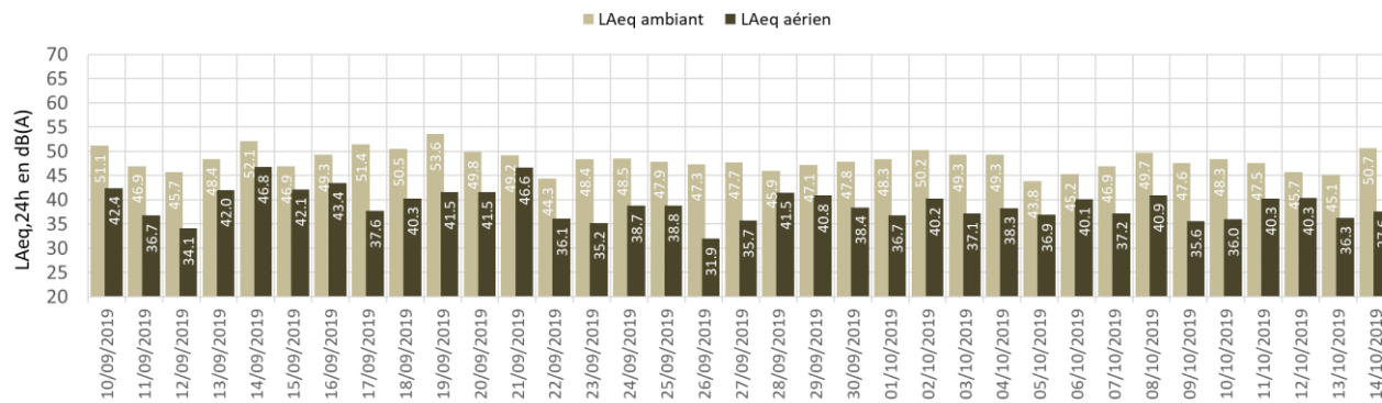
Évolution journalière du LAeq,24h - MONTEREAU
