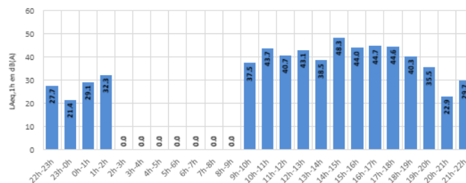
Distribution des LAMax - par périodes réglementaires - MONTEREAU Samedis - Configuration Ouest
