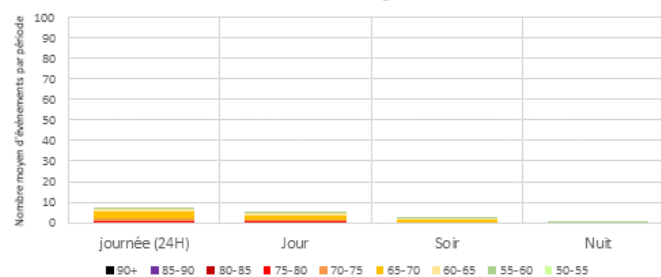
Distribution des SEL - par périodes réglementaires - RUBELLES Jours ouvrables - Configuration Est
