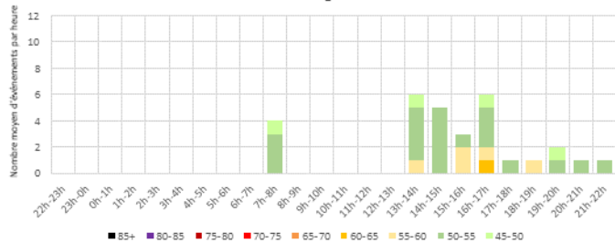
Distribution moyenne horaire des LAmx - RUBELLES Dimanches - Configuration Est
