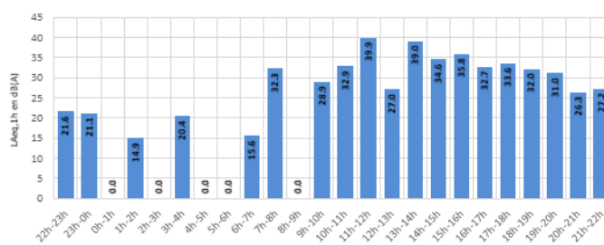
Niveau de bruit aérien - LAeq,1h - RUBELLES Tous jours confondus - Configuration Ouest
