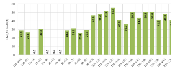
Distribution des LAMax - par périodes réglementaires - FOURCHES Samedis - Configuration Est
