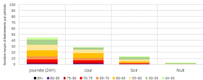
Distribution des LAmx - par périodes réglementaires - FOURCHES Tous jours confondus - Configuration Ouest
