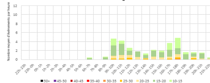
Distribution des émergences - par périodes réglementaires - MONTEAU Jours ouvrables - Configuration Est
