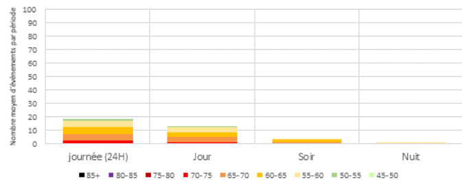
Distribution des LAmax - par périodes réglementaires - REAU Tous jours confondus - Configuration Est
