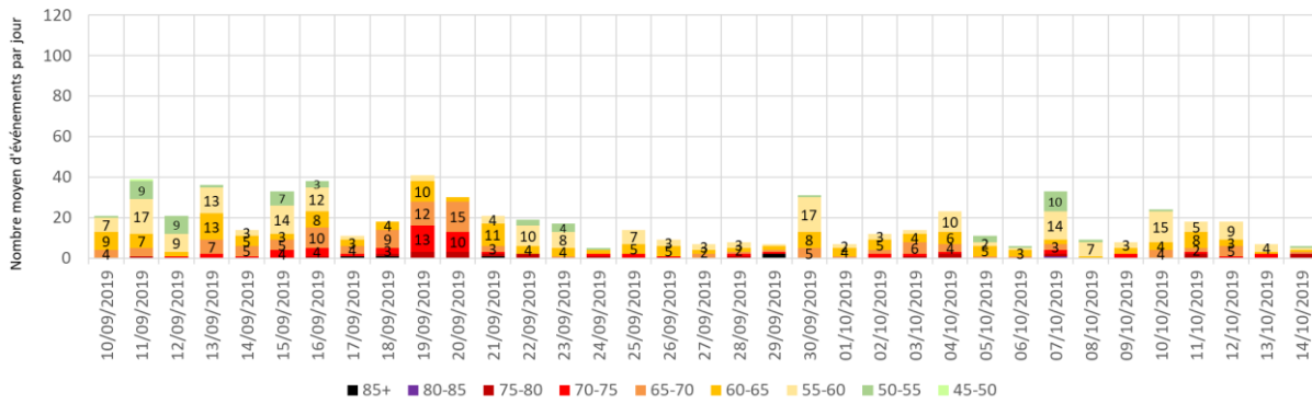
Distribution quotidienne (sur 24 heures) du LAmax des événements aériens - REAU
