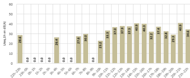
Niveau de bruit aérien - LAeq,1h - RUBELLES Samedis - Toutes configurations
