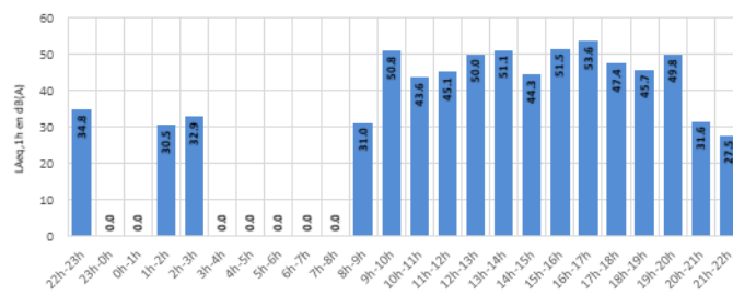
Distribution des LAMax - par périodes réglementaires - FOURCHES Samedis - Configuration Ouest
