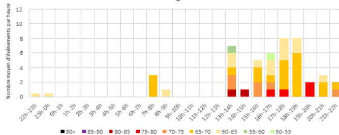
Distribution moyenne horaire des SEL - FOURCHES Dimanches - Configuration Est
