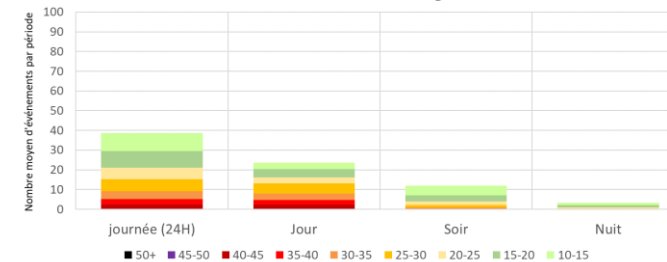
Distribution des émergences - par périodes réglementaires - FOURCHES Jours ouvrables - Configuration Est
