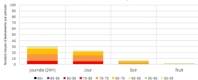
Distribution des SEL - par périodes réglementaires - MONTEREAU Jours ouvrables - Configuration Ouest
