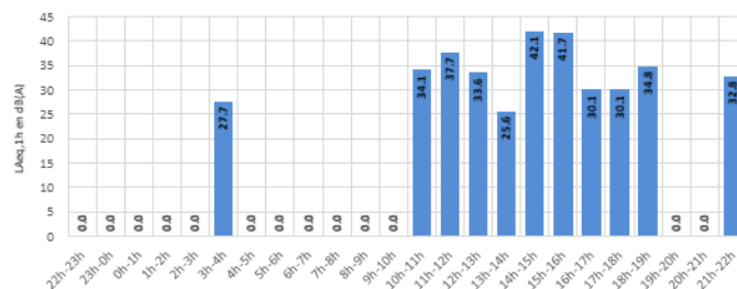
Distribution des LAMax - par périodes réglementaires - RUBELLES Samedis - Configuration Ouest
