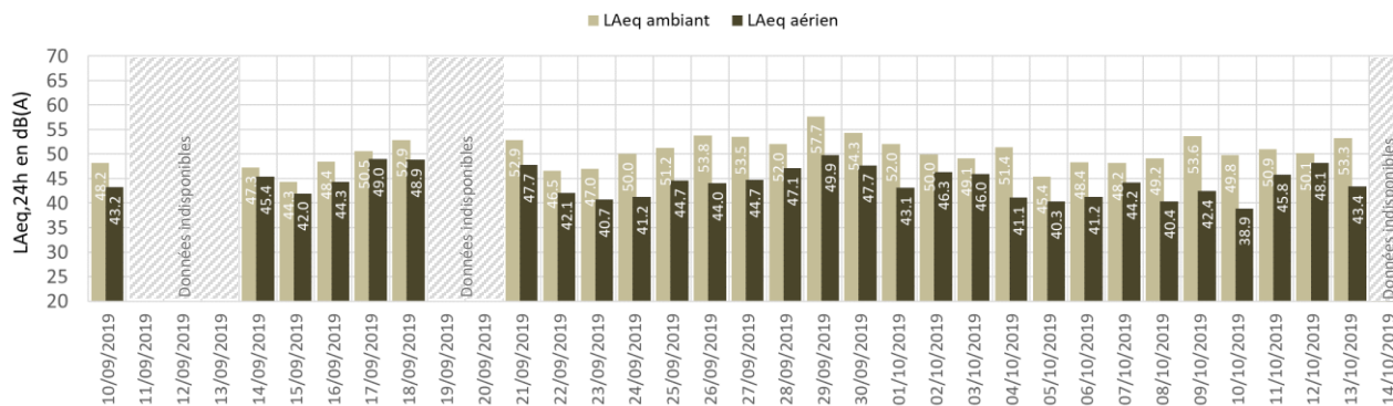
Évolution journalière du LAeq,24h - FOURCHES
