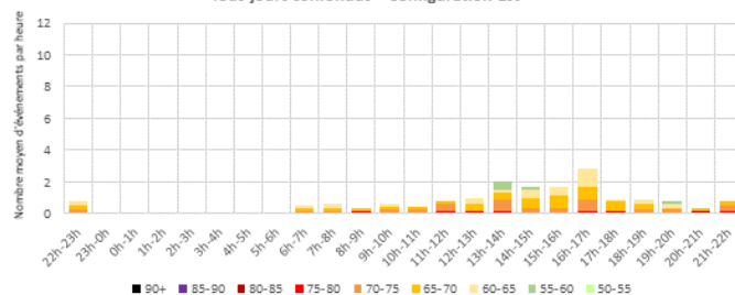
Distribution moyenne horaire des SEL - RUBELLES Tous jours confondus - Configuration Est
