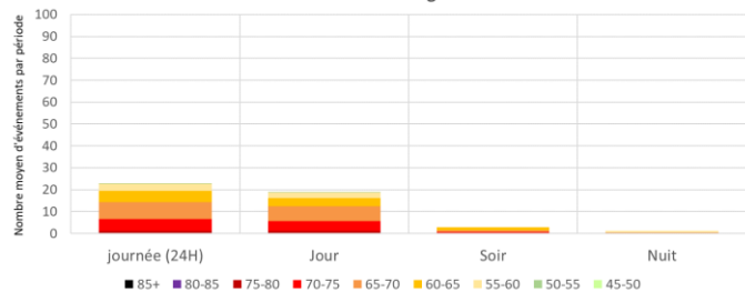
Distribution des LAmax - par périodes réglementaires - REAU Jours ouvrables - Configuration Est
