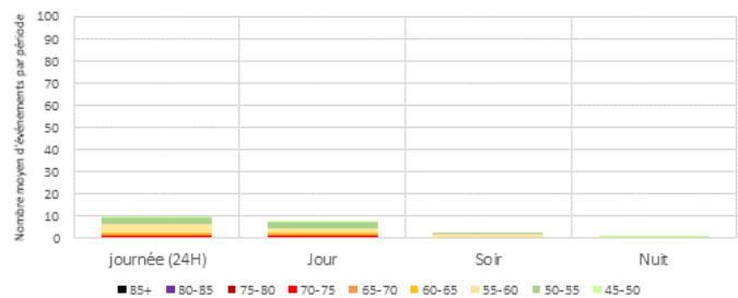
Distribution des LAmx - par périodes réglementaires - RUBELLES Samedis - Configuration Est
