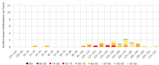
Distribution moyenne horaire des LAMax - REAU Samedis - Configuration Est
