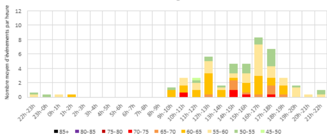
Distribution moyenne horaire des LAMax - MONTEREAU Samedis - Configuration Est
