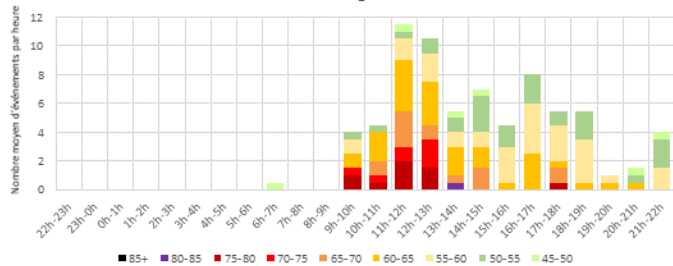
Distribution moyenne horaire des LAMax - MONTEREAU Samedis - Configuration Est
