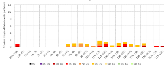
Distribution moyenne horaire des SEL - REAU Dimanches - Configuration Ouest
