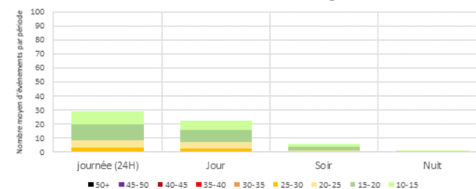
Distribution des émergences - par périodes réglementaires - MONTEREAU Jours ouvrables - Configuration Ouest
