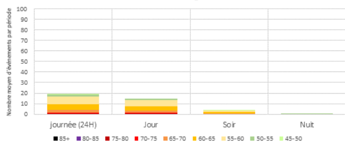
Distribution des LAmax - par périodes réglementaires - REAU Jours ouvrables - Configuration Est
