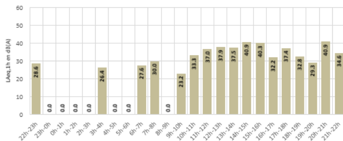
Niveau de bruit aérien - LAeq,1h - RUBELLES Dimanches - Toutes configurations
