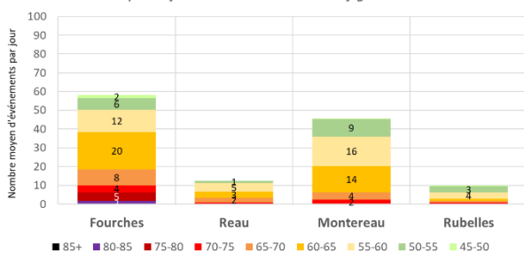
Distribution des L Max aéronefs sur la période de mesure Moyenne journalière - Samedis - Configuration OUEST
