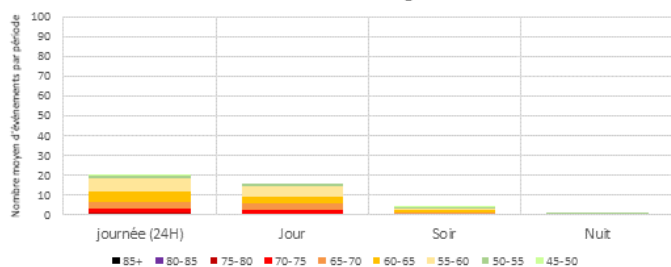
Distribution des LAmax - par périodes réglementaires - REAU Jours ouvrables - Configuration Ouest
