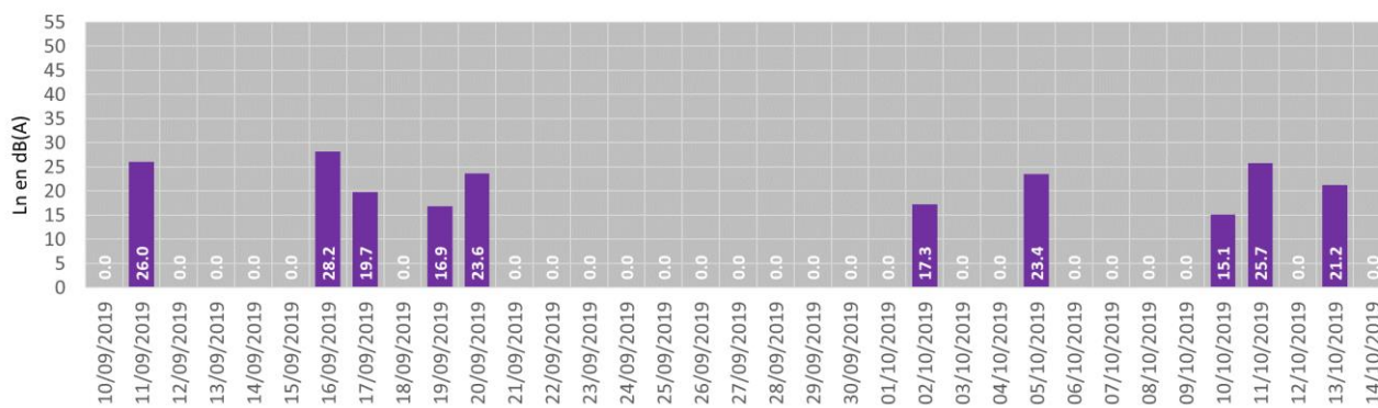
Évolution journalière du Ln aérien - RUBELLES
