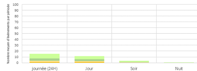
Distribution des émergences - par périodes réglementaires - REAU Tous jours confondus - Toutes configurations
