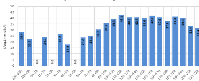
Niveau de bruit aérien - LAeq,1h - REAU Tous jours confondus - Configuration Ouest
