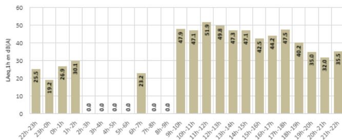
Niveau de bruit aérien - LAeq,1h - MONTEREAU Samedis - Toutes configurations
